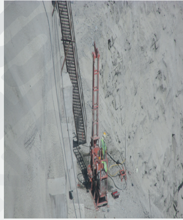
Yusufeli Barajı Havalı Delgi Çalışmaları
